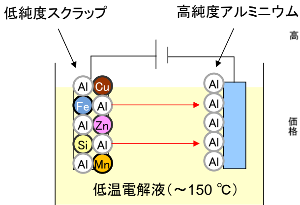
低温型電解法のイメージ図
